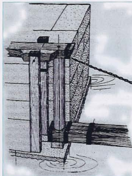
Particolare ricostruttivo del sistema di movimentazione della catena di chiusura dell'accesso al porto.
