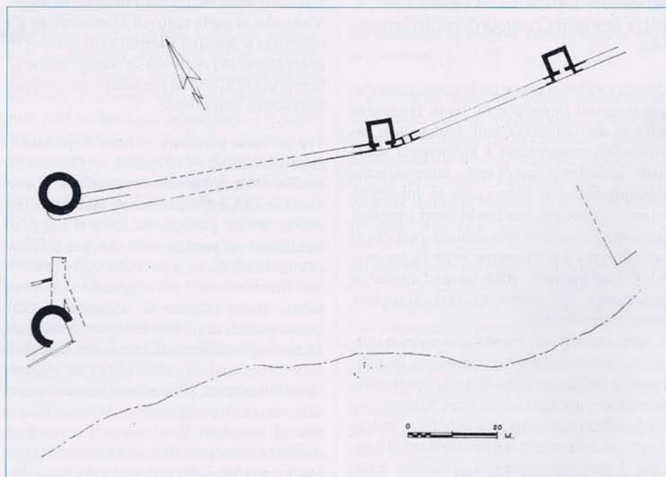
Halieis, planimetria della parte interna dell'area portuale (scavi 1968).
